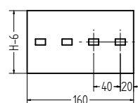
連接片 Connector
