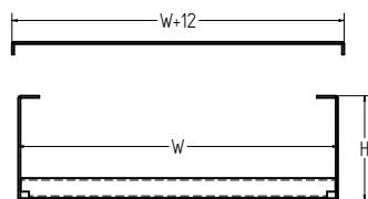
本體 Tray
